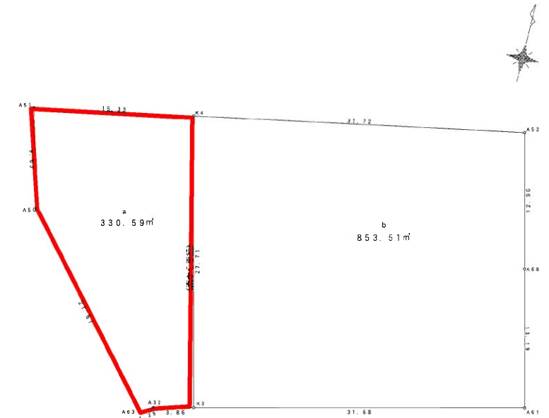
区画計画図
